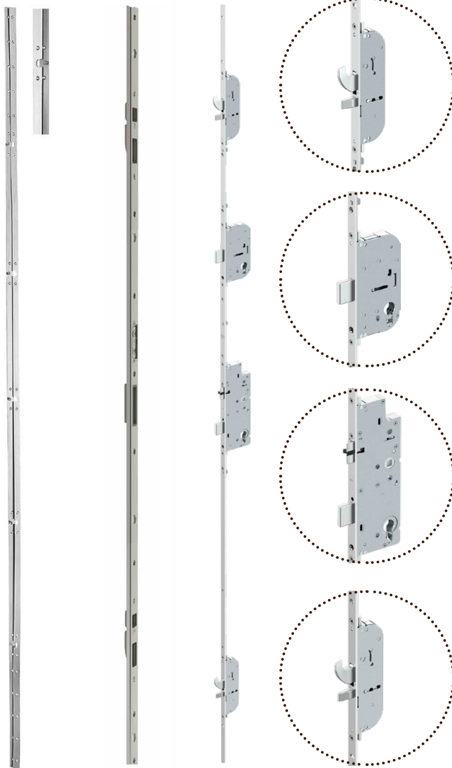
Listwa antywyważeniowa
